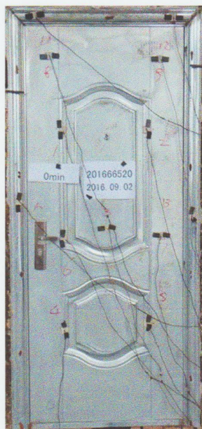
照片 1 耐火试验前试件情况
